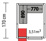
Kühlzelle Artikel-Nr.: 661031 Preis.: 1.999,00 €
