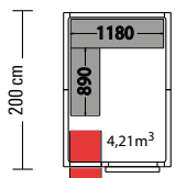
Kühlzelle Artikel-Nr.: 661032 Preis.: 2.195,00 €
