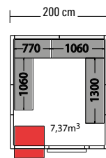
Kühlzelle Artikel-Nr.: 661040 Preis.: 3.048,00 €
